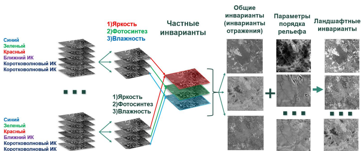
Рисунок 2 Алгоритм получения ландшафтных инвариантов на основе МДДЗ и ЦМР
