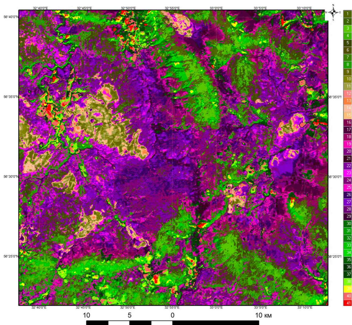
Рисунок 4 Классификация ландшафтных инвариантов (1 - 8 класс – хвойно-мелколиственные леса, 9 - 15 класс – верховые болота, 16 - 29 класс – мелколиственно-хвойные и хвойные леса, 30 – 39 класс – мелколиственные леса, 39 – 41 класс – луга, сенокосы, селитебные земли)
